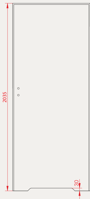
Podcięcie
