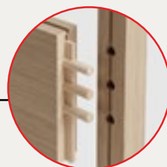
Moduły łączone za pomocą drewnianych kołków i warstwy kleju
