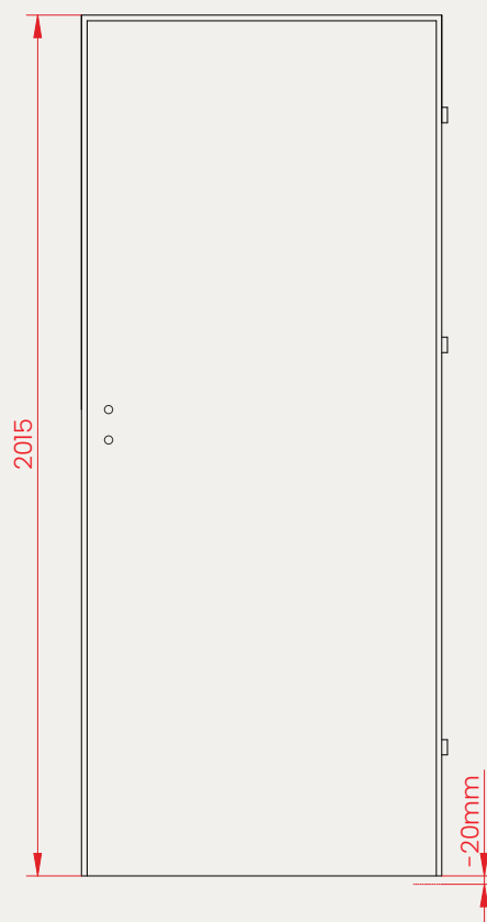
Podcięcie rekuperacyjne
